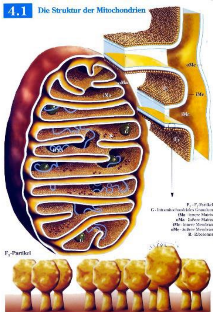
Querschnitt unseres Zellkraftwerks
