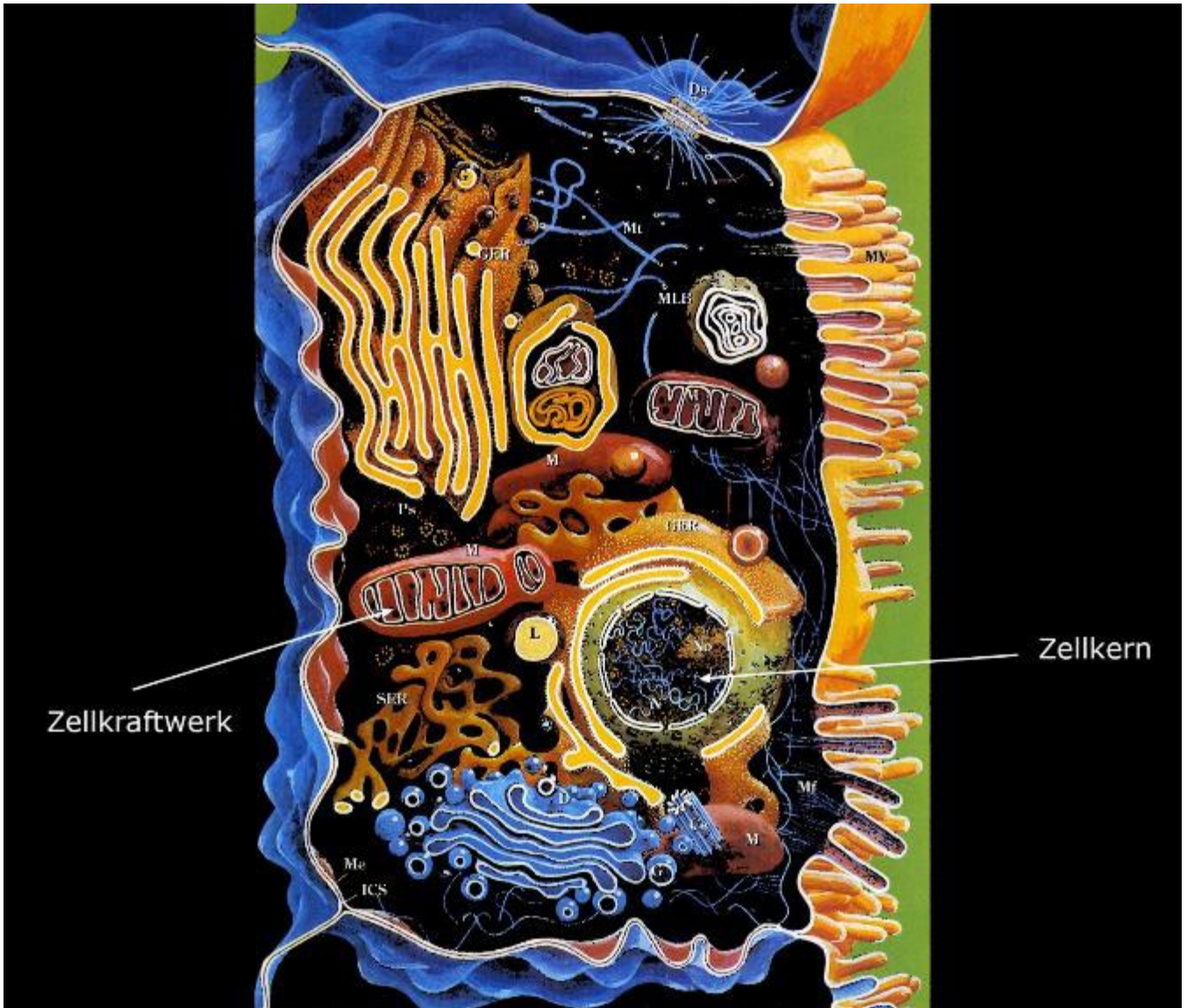
Zell Querschnitt mit Darstellung der Zell Organe
